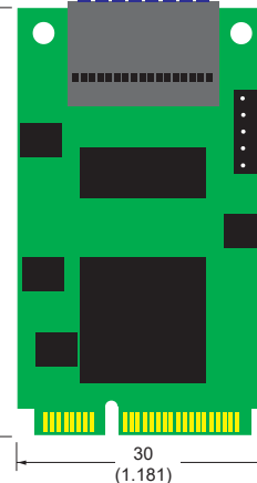
PIXCI® EB1MINI-G-S (SDR) PIXCI® EB1MINI-G-M (MDR)
